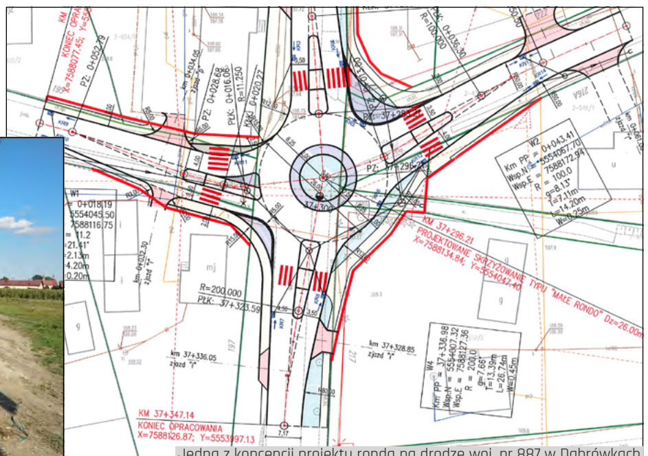
Jedna z koncepcji projektu ronda na drodze woj. nr 887 w Dąbrówkach
